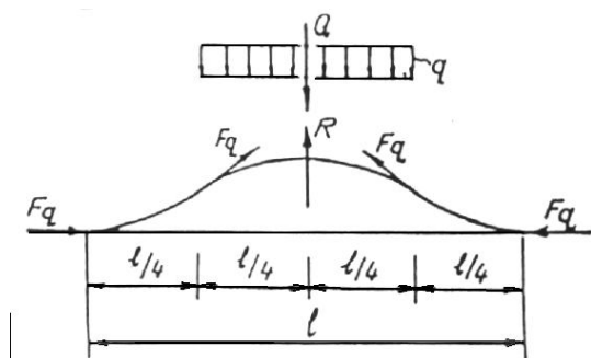
Fig. 3. Calculul forței F_q
